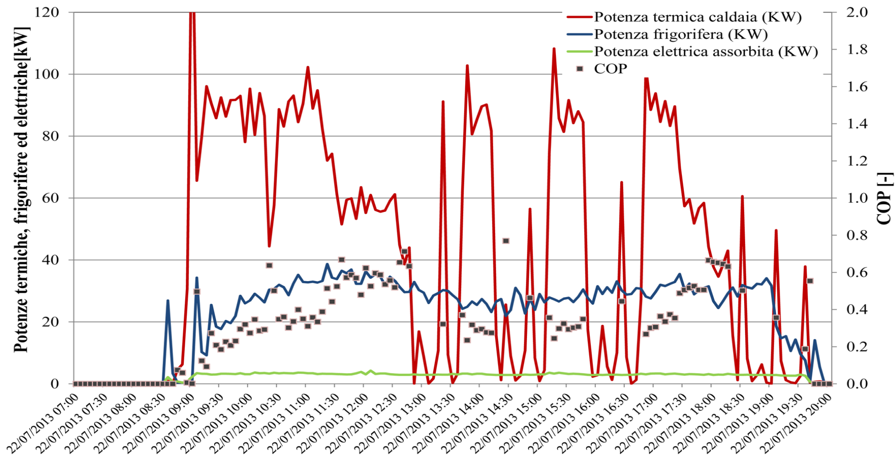
Grafico Potenze (kW) - 22 Luglio 2013
