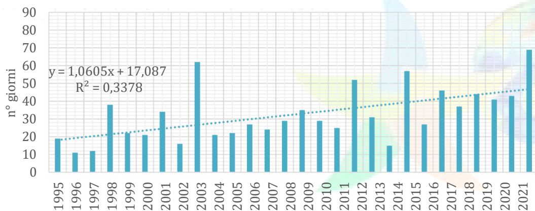
Indici climatici : Notti tropicali (TR20)
