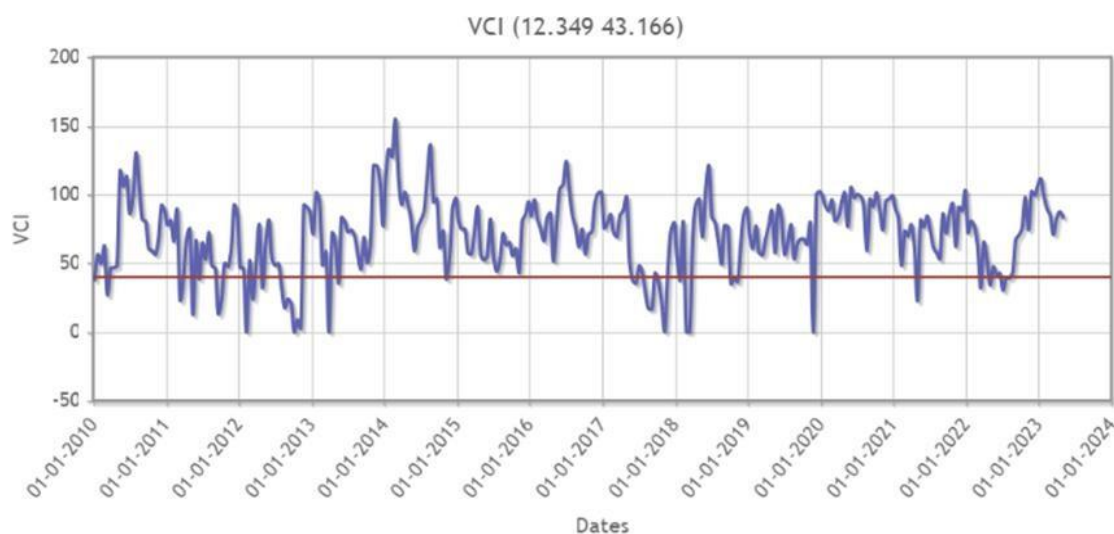
Figura 25: Estratto dell'indicatore VCI. Fonte: Drought Observatory CNR IBE
