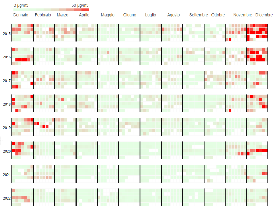
Figura 15: Stazione di Perugia Parco Cortonese, valore della media 24h di PM 2,5 (fonte: ARPA Umbria)
