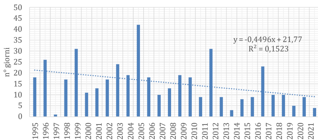
Indici climatici: Giorni con gelo (FD0)
