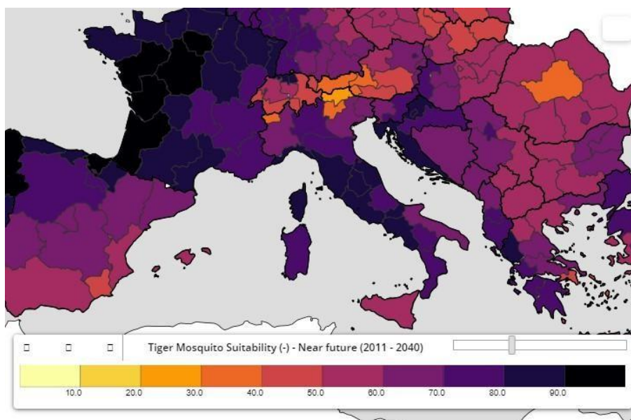
Figura 27: Indice di idoneità climatica alla zanzara tigre - scenario RCP4.5 [18].
