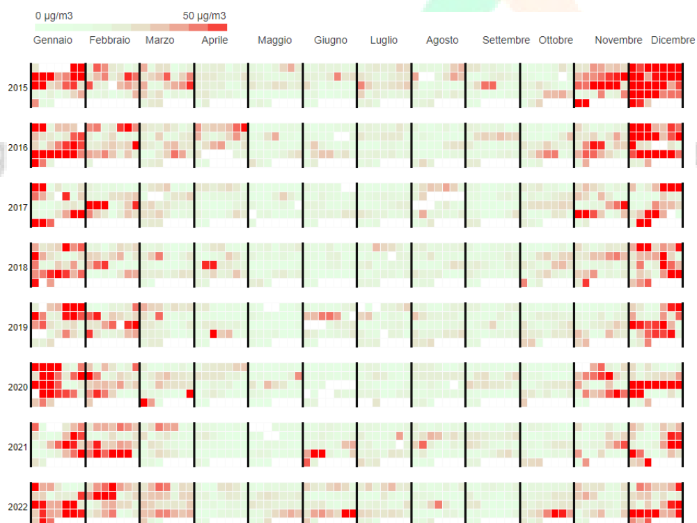
Figura 10: Stazione di Perugia Ponte S. Giovanni, valore della media 24h di PM10 (fonte: ARPA Umbria)
