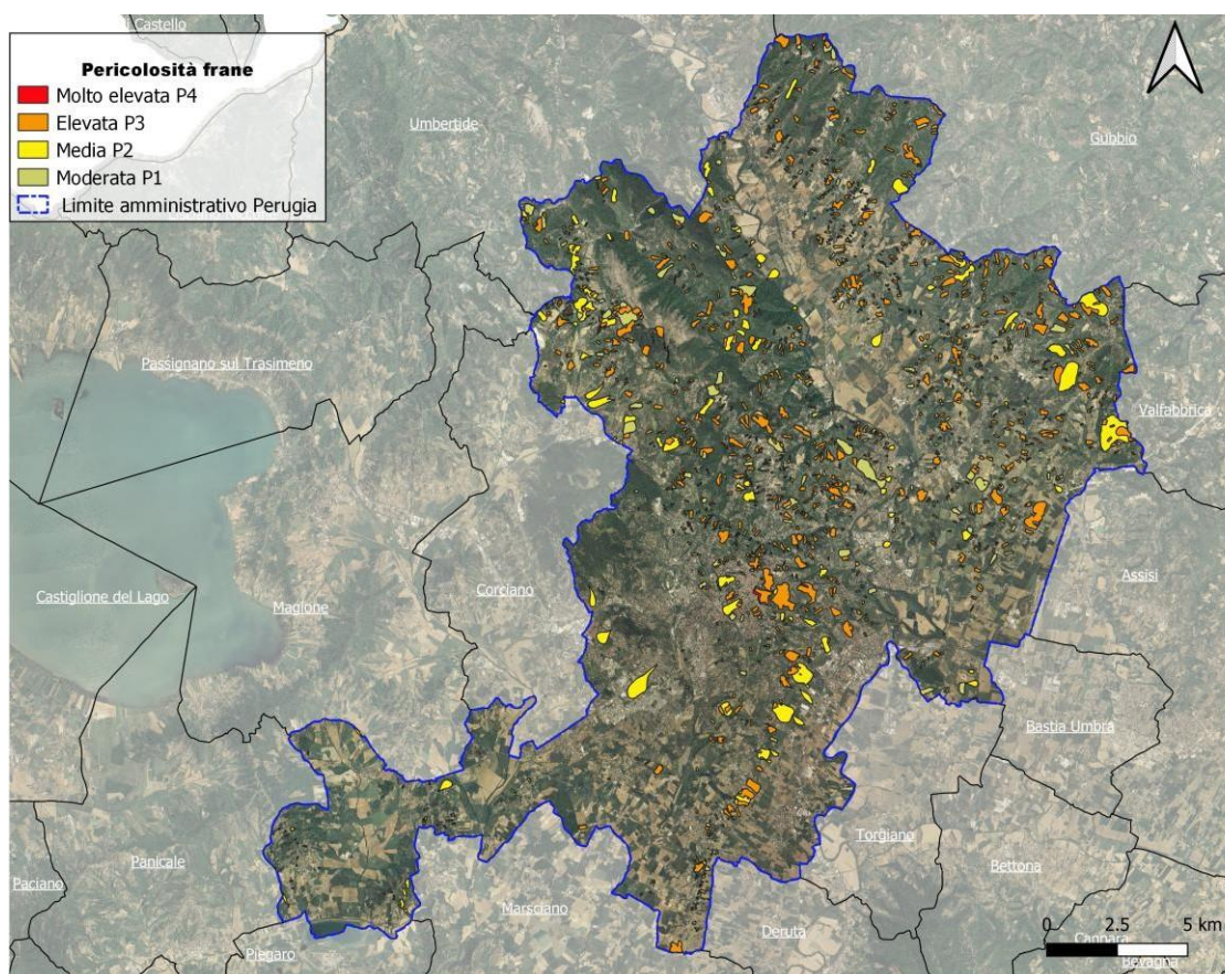
Figura 20: Individuazione delle aree più suscettibili agli impatti causati da frane e indicazione del livello di pericolosità. Fonte: elaborazione su QGis dei dati ISPRA [13].
