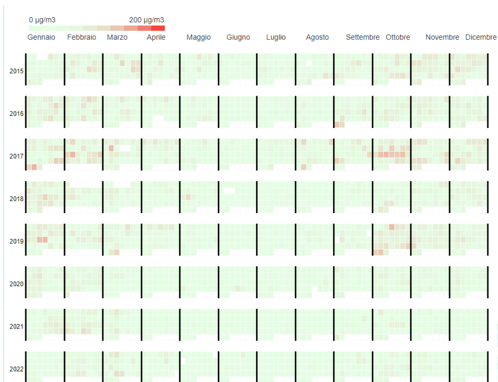
Figura 18: Stazione di Perugia Ponte S.Giovanni, medie dei valori orari di NO 2 (fonte: ARPA Umbria)
