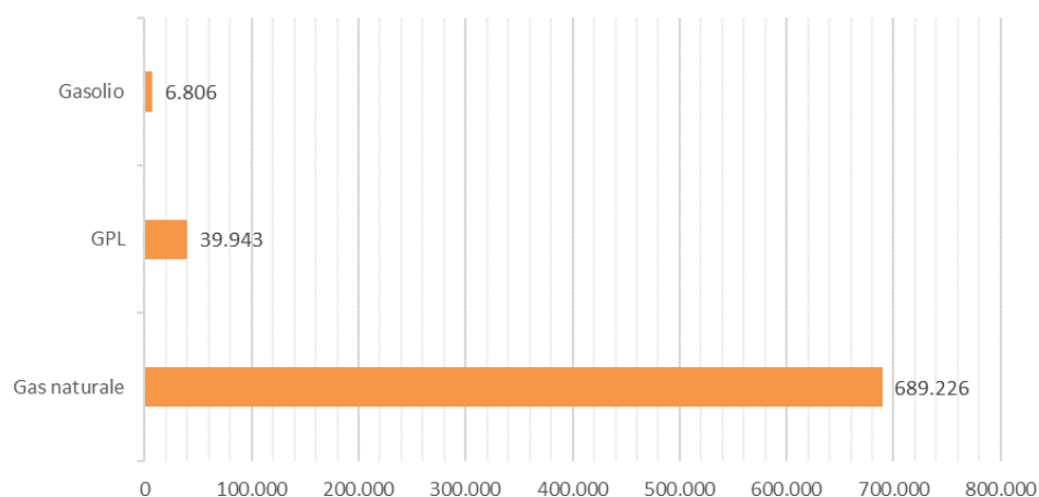
Grafico 19 - Consumi termici settore residenziale (2015).
