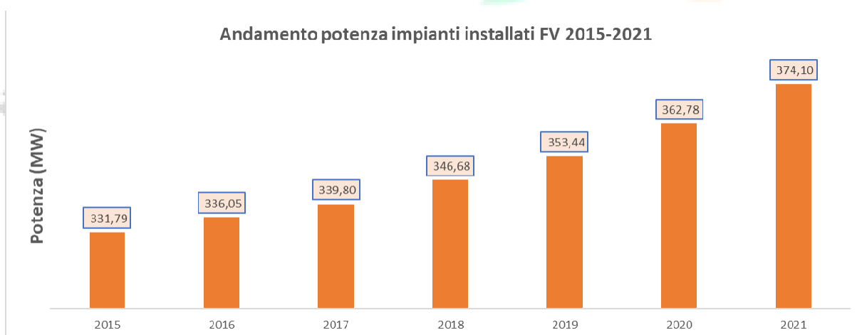
Grafico 6 - Andamento della potenza degli impianti fotovoltaici installati nella provincia di Perugia. (Fonte: Atlaimpianti GSE)
