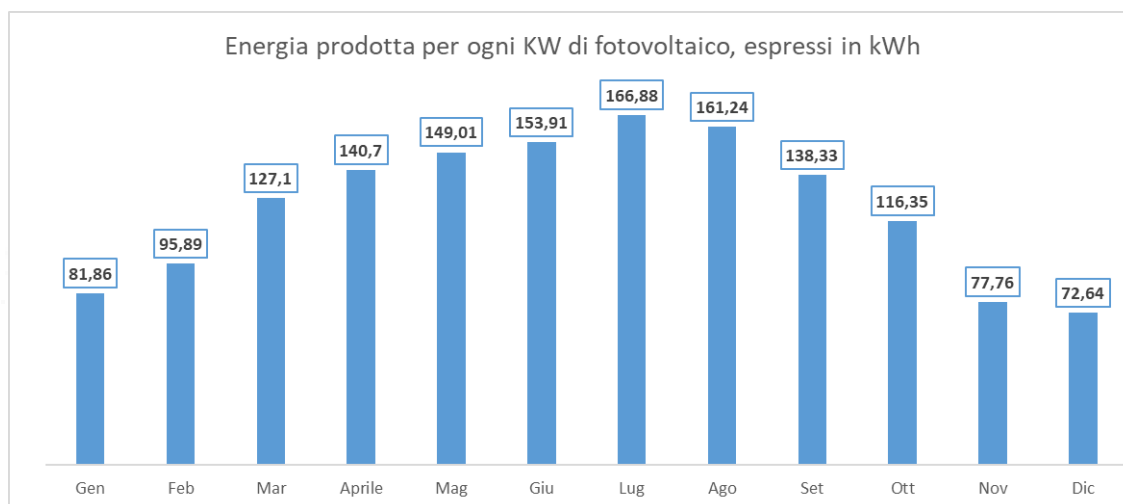
Grafico 4 - Producibilità media annua per ogni kW di potenza.
