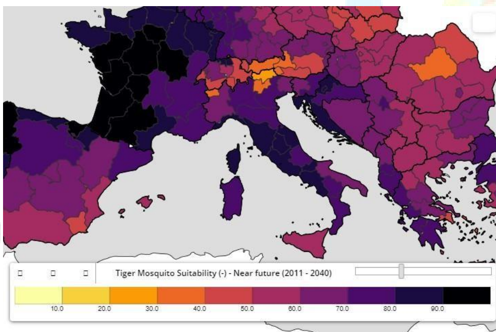
Figura 28: Indice di idoneità climatica alla zanzara tigre - scenario RCP8.5 [18].
