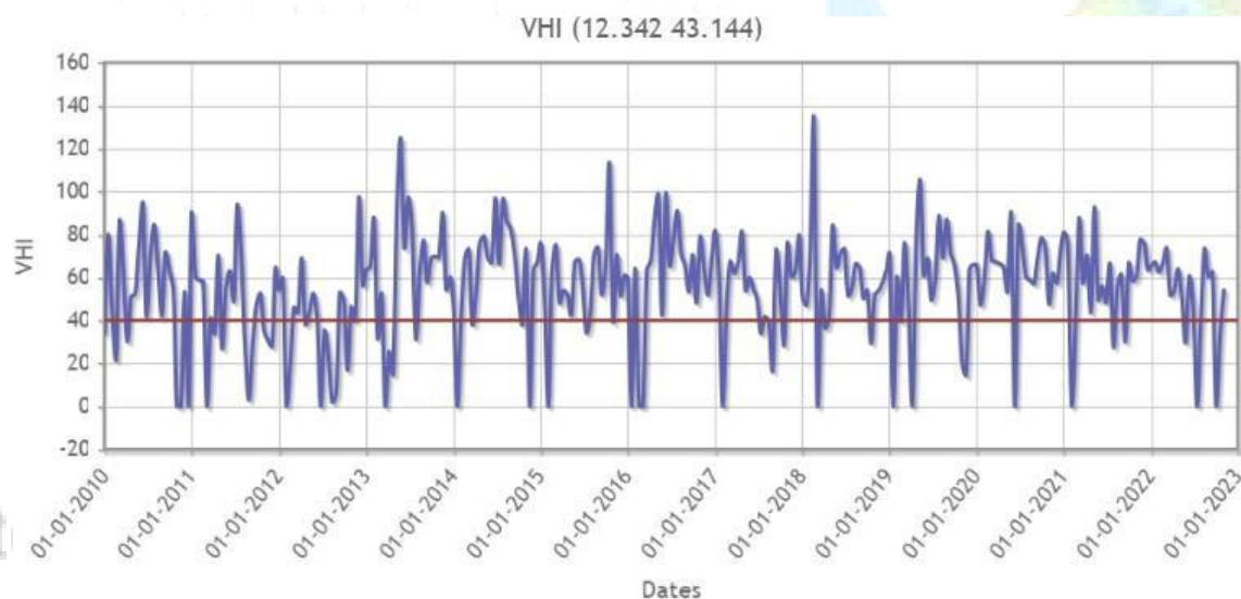
Figura 26: Estratto dell'indicatore VHI. Fonte: Drought Observatory CNR IBE
