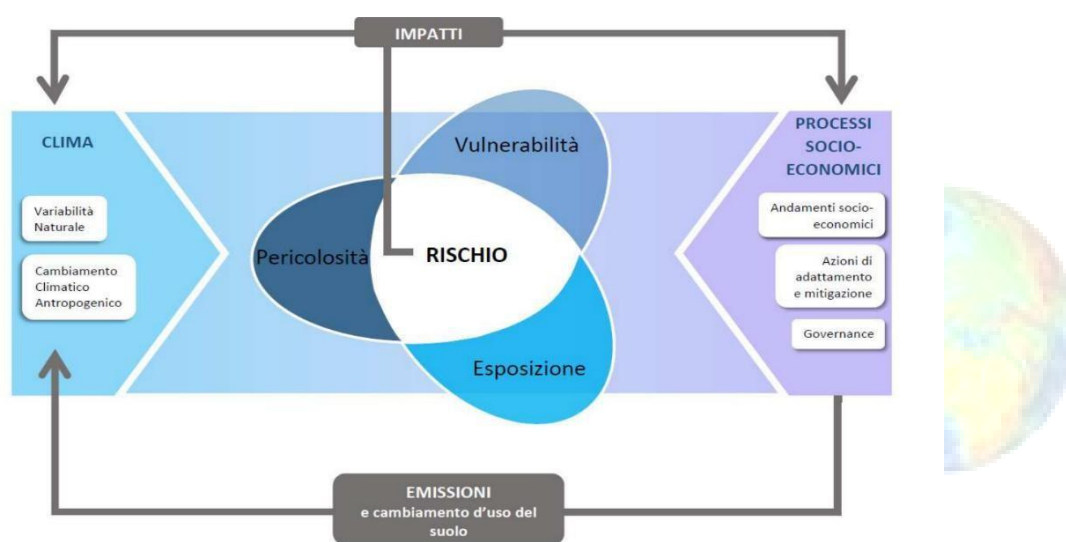
Figura 17 - Componenti fondamentali per la determinazione del rischio legato ai cambiamenti climatici. Fonte: Panel Intergovernativo sui Cambiamenti Climatici (IPCC, 2014)
