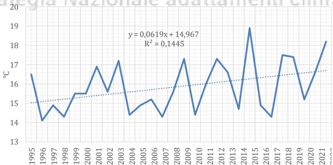
Indici climatici: Massimo delle temperature minime (TNx)
