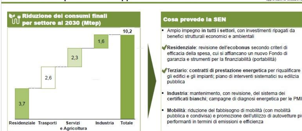
Figura 5 – Obiettivo di riduzione dei consumi finali (Fonte: SEN 2017).
