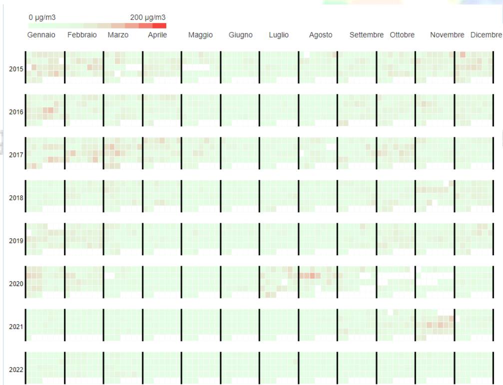
Stazione di Perugia Parco Cortonese, medie dei valori orari di NO 2 (fonte: ARPA Umbria)
