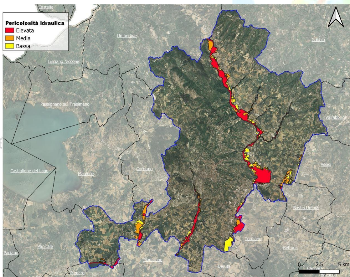
Figura 2120: Individuazione delle aree che ricadono in aree a pericolosità idraulica. Fonte: elaborazione su QGIS dei dati ISPRA sulla mosaicatura delle aree a pericolosità idraulica [20].
