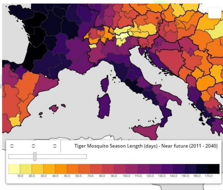
Figura 30: Durata della stagione di idoneità alla zanzara tigre - scenario RCP8.5 [18].
