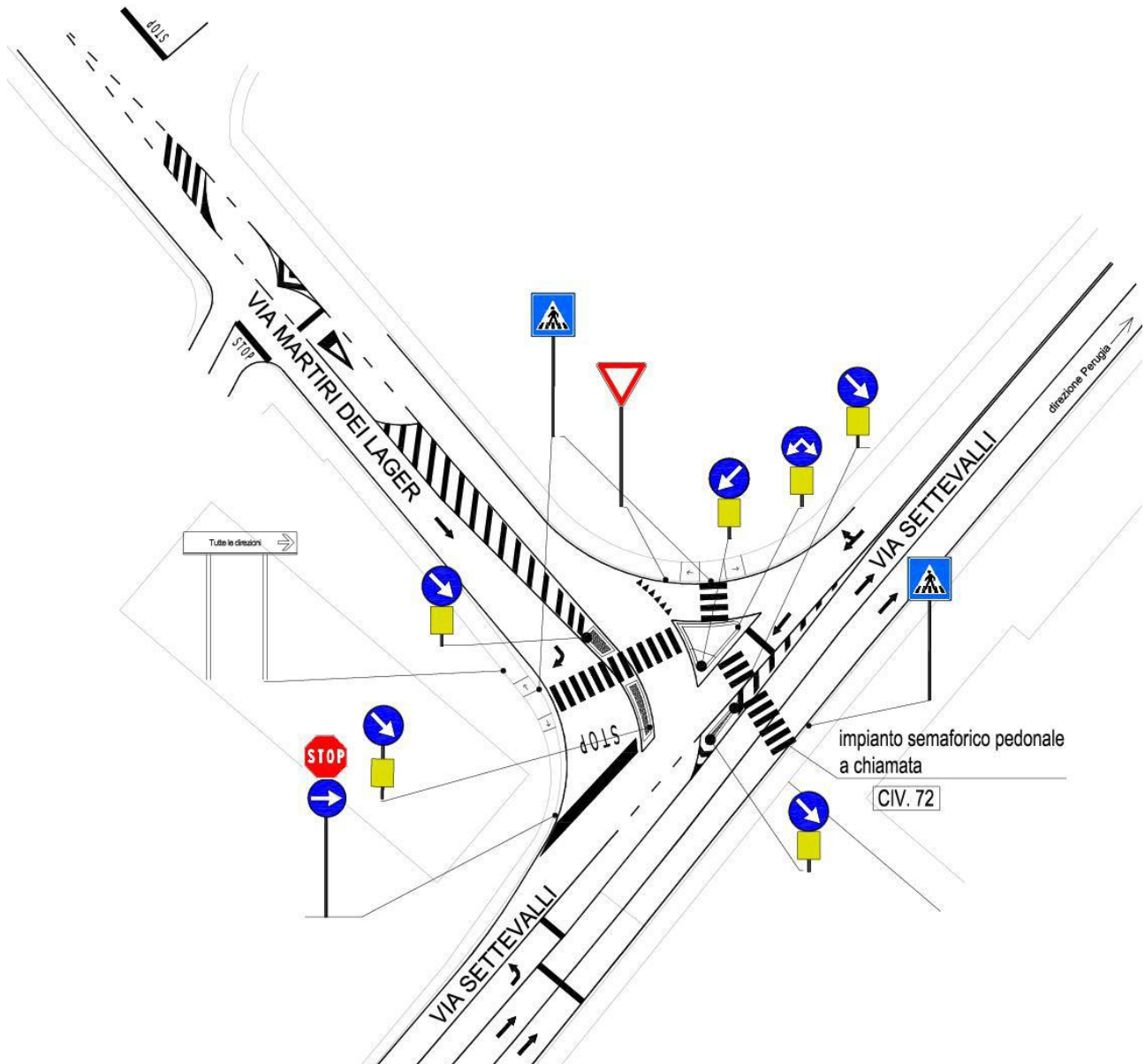
Fig. 1 - Planimetria
