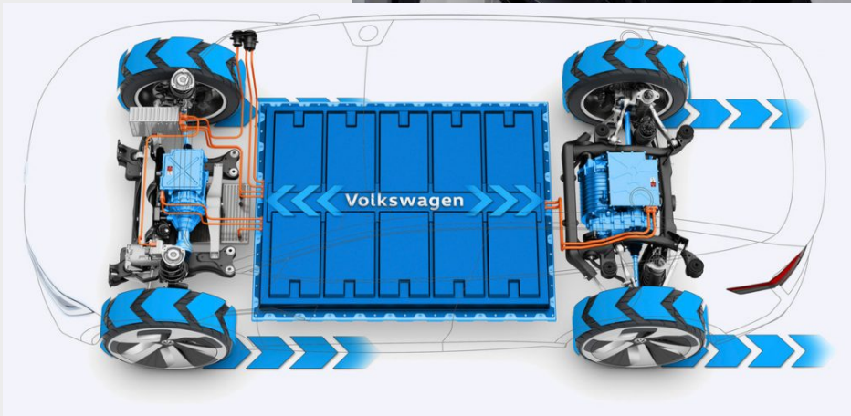
Flüssigkeitsgekühlte Lithium-Ionen-Batterie mit 95 kWh Liquid-cooled lithium-ion battery with 95 kWh
